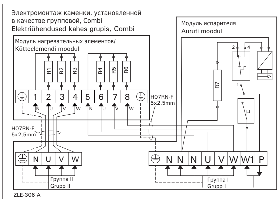
Рисунок 10. Электромонтаж Joonis 10. Elektriühendused
