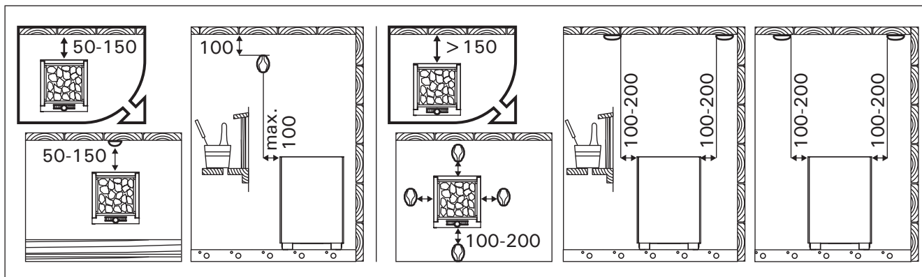
Kuva 7. Lämpöanturin asentaminen (mitat millimetreinä) Bild 7. Montering av temperaturgivaren (mått i millimeter)
