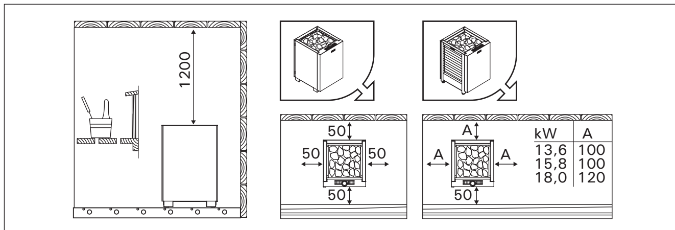
Kuva 5. Kiukaan minimisuojaetäisyydet (mitat millimetreinä) Bild 5. Minimum säkerhetsavstånd (måttan i millimeter)
