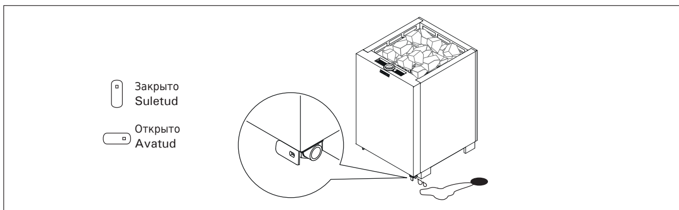
Рисунок 2. Опорожнение резервуара для воды Joonis 2. Veepaagi tühjendamine
