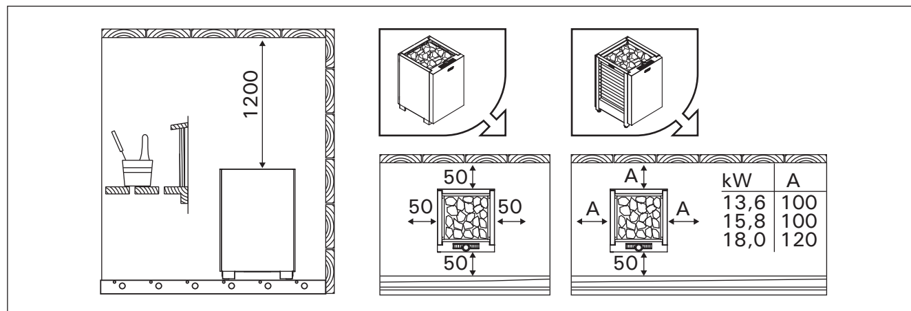
Рисунок 5. Расстояния безопасности (все размеры приведены в миллиметрах) Joonis 5. Kerise miinimum ohutuskaugused (kõik mõõtmised millimeetrites)
