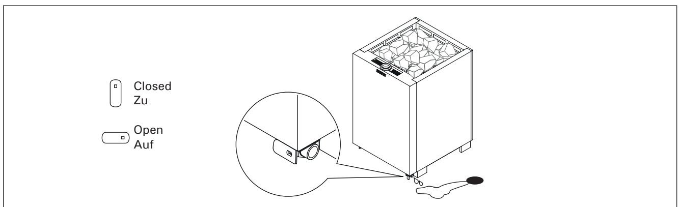
Figure 2. Draining the water reservoir Abbildung 2. Leeren des Wassertanks
