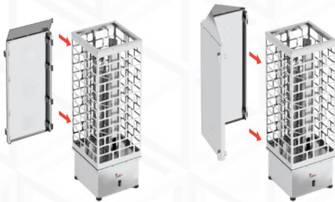
Пристенная установка с защитным ограждением
